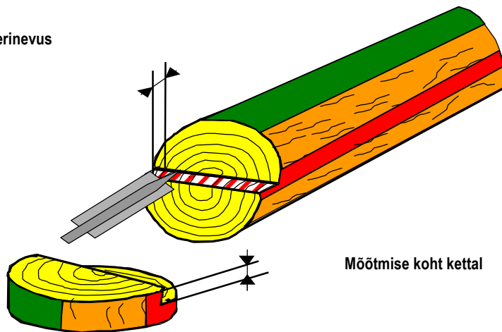
Joon 23: Lõiketaseandite erinevus mõõdetakse palgil ja kettal
